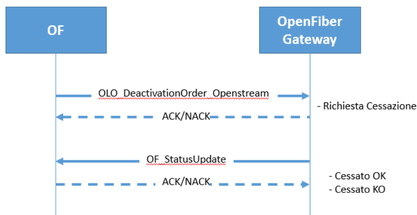
Figura 2: Cessazione servizio OpenStream
