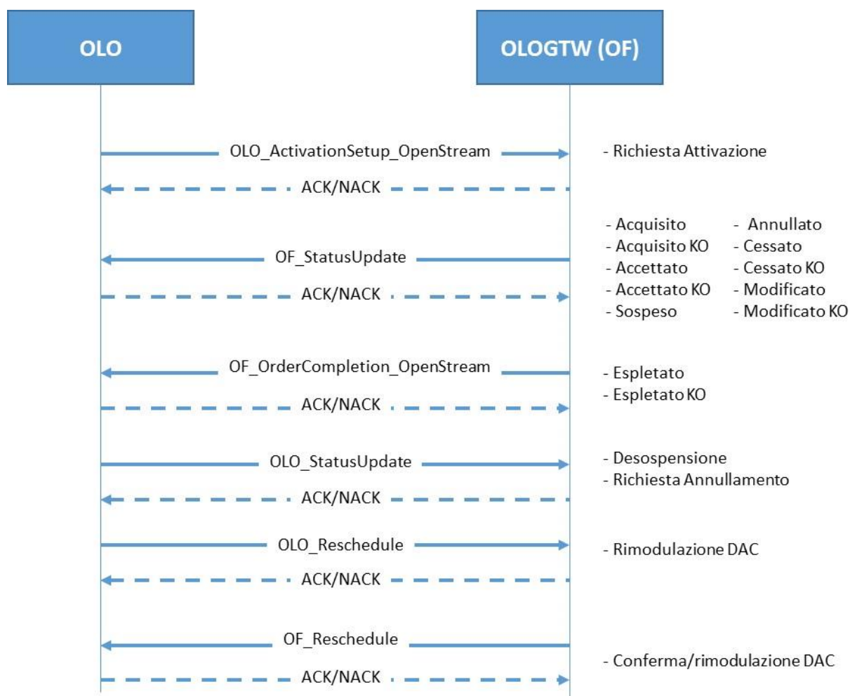
Figura 1: Attivazione servizio Open Stream
